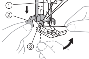
① Иголдержатель ② Рычажок нитевдевателя ③ Направляющая
