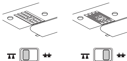
► Гребенки транспортера опущены.
