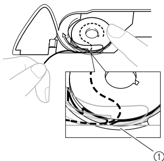
① Пружина регулировки натяжения нити
