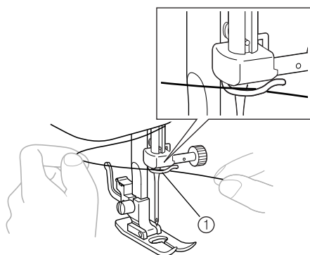
① Нитенаправитель игловодителя
