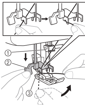
① Игольдержатель ② Рычажок нитевдевателя ③ Направляющая
