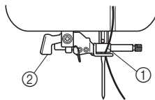
1 Иглодержатель 2 Рычажок нитевдевателя
